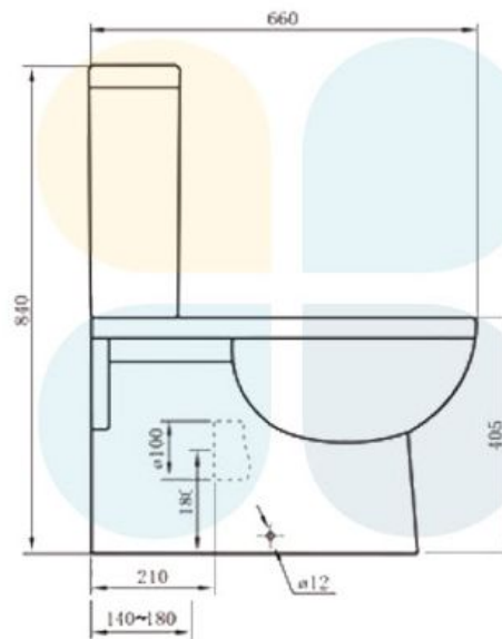
houston toilet suite TP-1008
